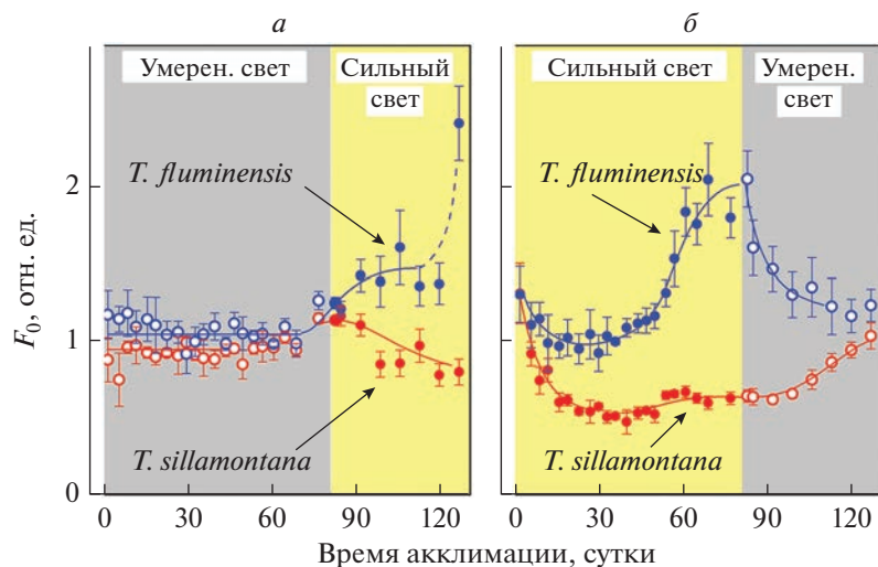
Рис. 3. Динамика изменений параметра F_0 кривой быстрой индукции флуоресценции, измеренного в листьях T. fluminensis и T. sillamontana , произрастающих в условиях освещения “сильным” и “умеренным” светом. Вертикальные линии — стандартное отклонение от средних значений, полученных для n = 4-8 измерений.
