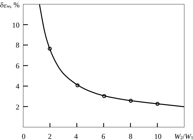
Рис. 7. Относительная среднеквадратичная погрешность \delta_{Ew} в зависимости от отношения мощностей тепловыделений W_2/W_1 Результаты и обсуждение
