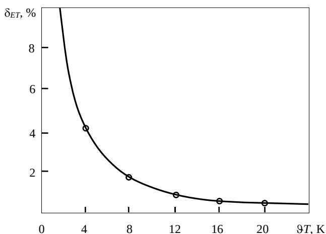
Рис. 6. Относительная среднеквадратичная погрешность \delta_{ET} в зависимости от разности температур \Delta T в двух экспериментах
