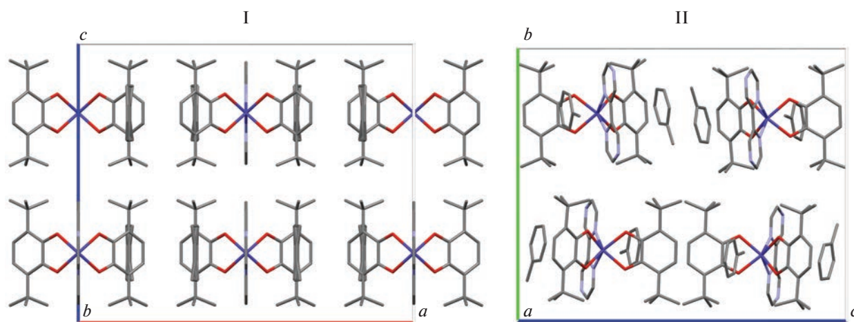
Рис. 2. Вид сбоку на элементарные ячейки комплексов I и II.
