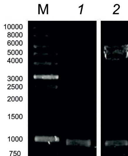
Рис. 1. Электрофореграмма продуктов клонирования генетической кассеты “биназа–барстар” в вектор pTurboGFP-C: М – маркер длин ДНК 1 кб (Сибэнзим, Россия); 1 – ПЦР-продукт “биназа–барстар”; 2 – полученная генетическая конструкция pTurboGFP-Bi-Brst, рестрицированная по сайтам XhoI и BamHI.
