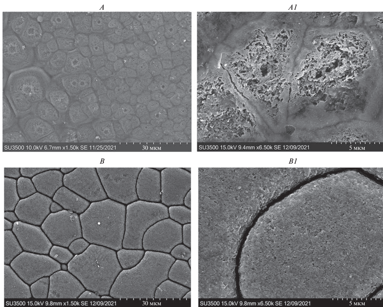
Рис. 3. СЭМ-изображения призматического слоя ростового края раковины диплоидных устриц Crassostrea gigas : A , AI – внутренняя сторона правой створки; B , BI – внутренняя сторона левой створки.
