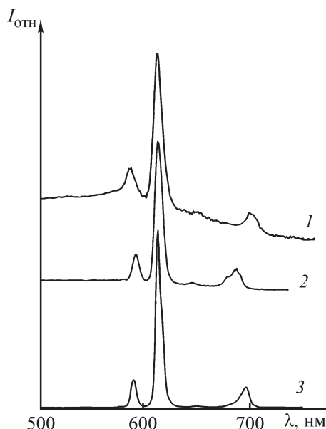
Рис. 2. Спектры люминесценции полиэтилена высокого давления с добавками соединений: 1 — \text{Eu(Quin)}_3 \cdot \text{gu} \cdot 2\text{H}_2\text{O} , 2 — \text{Eu(Quin)}_3 \cdot \text{dmf} \cdot 2\text{H}_2\text{O} , 3 — \text{Eu(Quin)}_3 \cdot \text{bt} \cdot 2\text{H}_2\text{O} .
