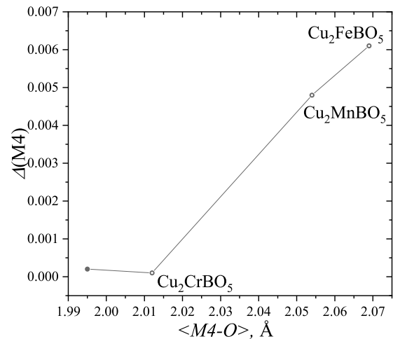
Рис. 2. Зависимость параметра октаэдрического искажения \Delta от среднего межионного расстояния позиции M4 для семейства людовгитов \text{Cu}_2\text{MBO}_5 ( M = \text{Cr}, \text{Fe}, \text{Mn} ). Темным кружком обозначено значение \Delta для \text{Cu}_2\text{CrBO}_5 из работы [8]
