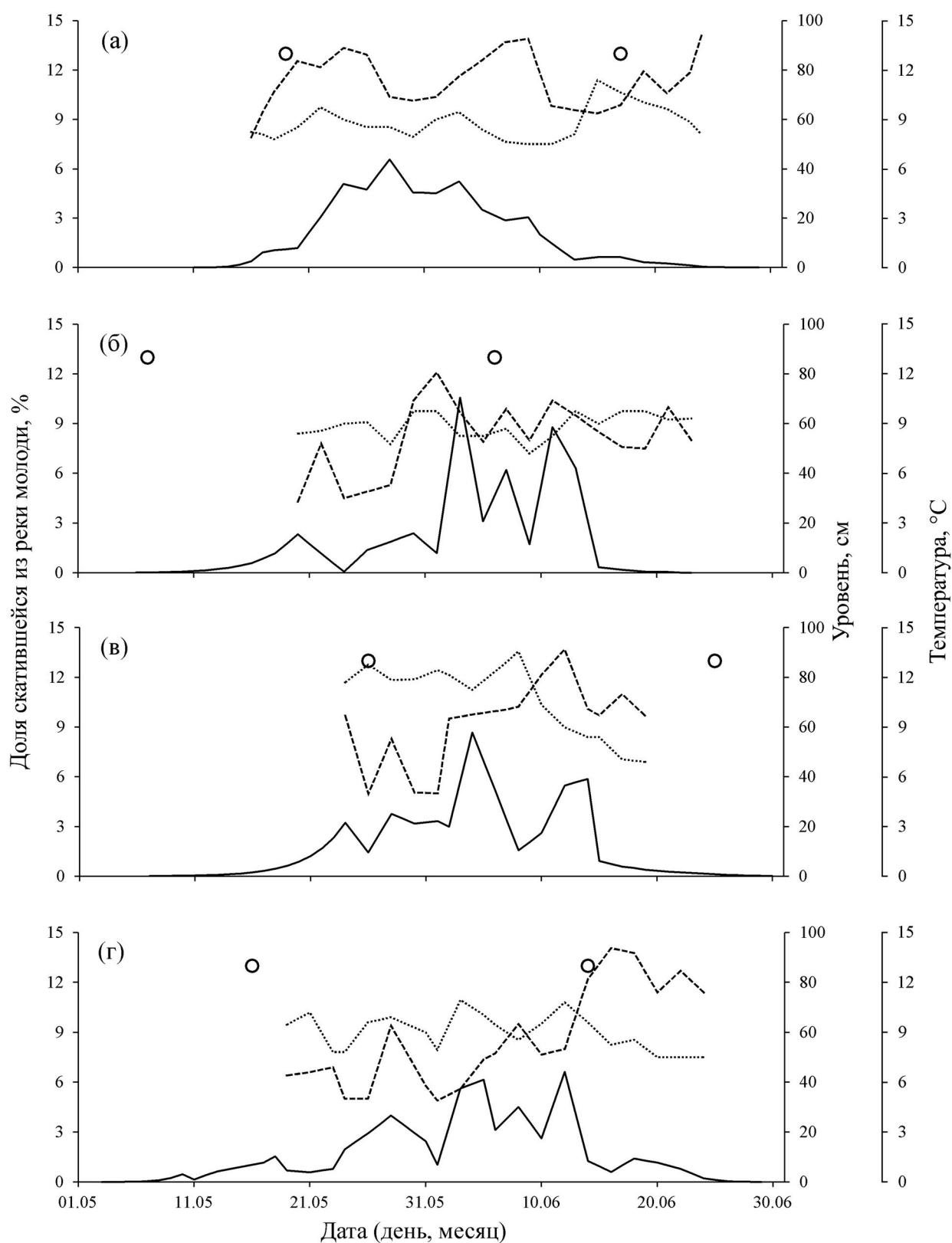
Рис. 3. Динамика покатной миграции молоди горбуши Oncorhynchus gorbuscha , температуры и уровня воды в р. Лазовая в мае–июне 2019 (а), 2020 (б), 2021 (в) и 2022 (г) гг. Здесь и на рис. 4, 5: обозначения см. на рис. 2.
