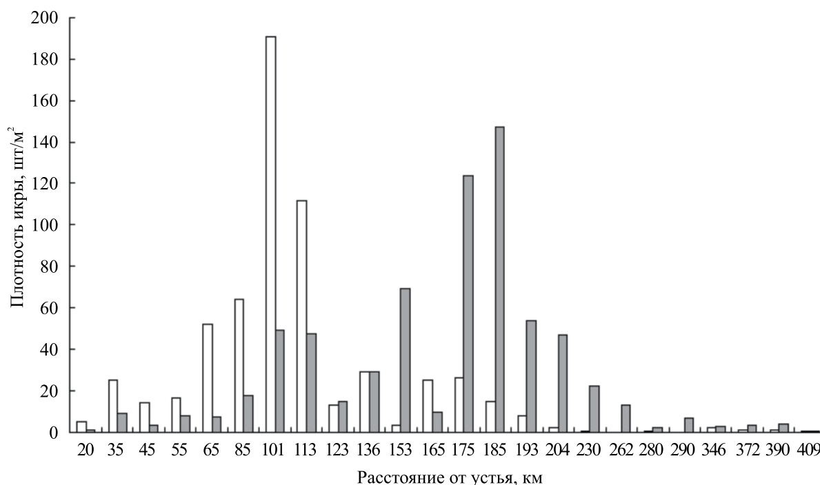
Рис. 4. Распределение икры байкальского омуля Coregonus migratorius в р. Селенга в 1984–2019 гг.: (□) – многоводные, (■) – маловодные годы. Максимальное количество икры на участке может не совпадать с максимумом плотности икры из-за разной площади участков нерестилищ: например, пик плотности икры может приходиться на определённый километр, пик же количества икры – на другой.
