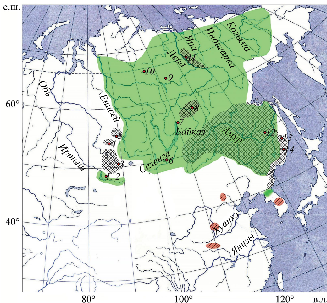
Рис. 1. Карта распространения трёх форм ленка рода Brachymystax : (▨) – тупорылая, (■) – острорылая, (■) – циньлинская. Ленок из рек Тумень и Ялу (Северная Корея, Китай) отнесён к острорылой форме (пояснения см. в тексте). Места взятия выборок (●) острорылого и тупорылого ленков, использованных для аллозимного анализа: 1 – р. Кальд-жир, 2 – оз. Маркаколь, 3 – р. Пыжа, 4 – р. Мрассу, 5 – р. Большой Кемчуг, 6 – р. Селенга, 7 – оз. Фролиха, 8 – р. Куанда, 9 – р. Моркока, 10 – р. Виллой, 11 – р. Ундюлонг, 12 – р. Хор, 13 – реки бассейна Японского моря (Самарга, Единка, Венюковка) объединены в выборку Северное Приморье, 14 – р. Таёжная (Центральное Приморье).
