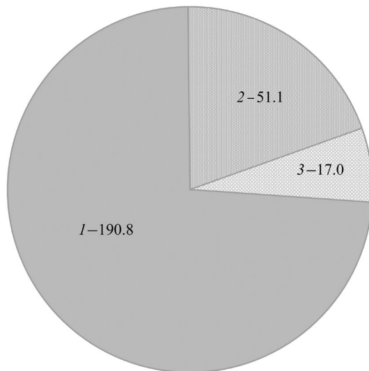
Рис. 6. Среднегодовое потребление (млн т) минтаем Gadus chalcogrammus гидробионтов (доминирующие группы) в эпипелагиали Берингова моря в 2011–2020 гг.: 1 – планктон (73.7%): Cooperoda (41.4%), Euphausiacea (20.7%), прочие (11.6%); 2 – нектон (19.7%): Pisces (17.5%), Decapodiformes (2.2%); 3 – бентос (6.6%): Decapoda (5.1%), прочие (1.5%).
