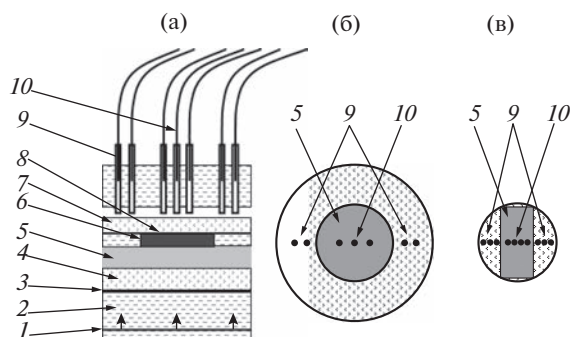
Рис. 1. Экспериментальная сборка.
