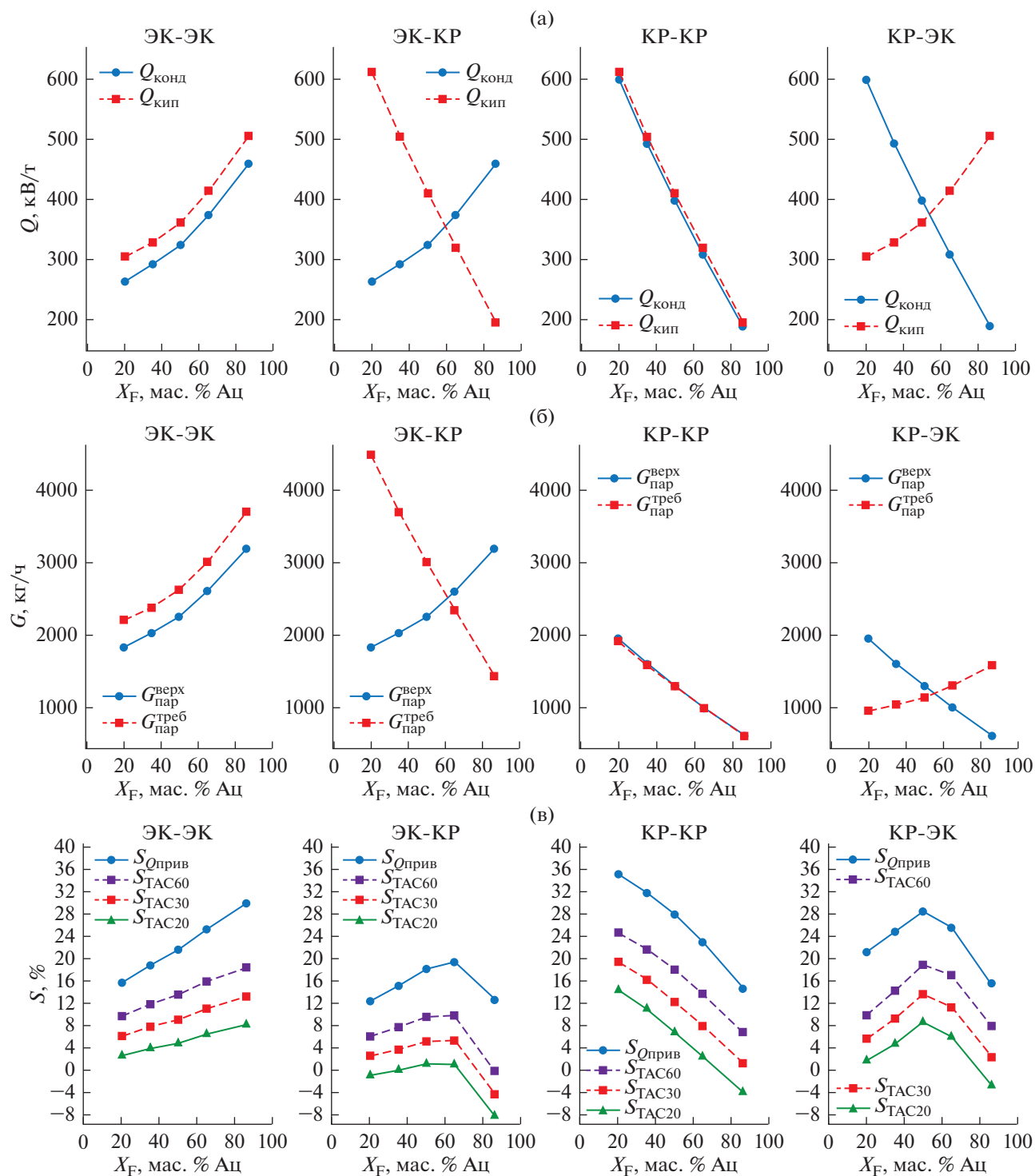
Рис. 3. Зависимости параметров и показателей схем ЭР смеси ацетон–метанол с ТН от состава исходной смеси: (а) нагрузки заменяемых кипяtilьника Q_{\text{кип}} и конденсатора Q_{\text{конд}} (источников и стоков тепла), (б) массовые расходы требуемого G_{\text{пар}}^{\text{треб}} и располагаемого G_{\text{пар}}^{\text{верх}} потоков пара, (в) показатели снижения годовых затрат S_{\text{TAC}} для сроков 20, 30 и 60 лет и приведенного энергосбережения S_{Q_{\text{прив}}} .
