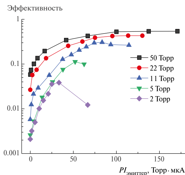
Рис. 4. Эффективность эвакуации ионов ^{219}\text{Rn} при напряжении катода -20 В для различных значений тока эмиттера и давления гелия.
