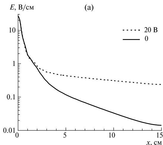
Рис. 3. Напряженность электрического поля (а) и плотность электронов (б) внутри ионного источника при давлении 25 \text{ Торр} и токе эмиттера 1 \text{ мкА} . Сплошная линия — распределение при нулевом потенциале на фольгах с нанесенным ураном. Штриховая линия — к фольгам приложен потенциал, возрастающий от 0 до 20 \text{ В} по мере удаления от катода. По оси абсцисс указано расстояние до катода.
