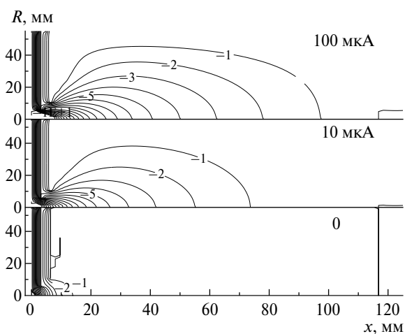
Рис. 2. Распределение потенциала внутри ионного источника, рассчитанное для различных токов эмиттера при давлении 50 \text{ Торр} . Числами показаны значения потенциала для эквипотенциальных линий.
