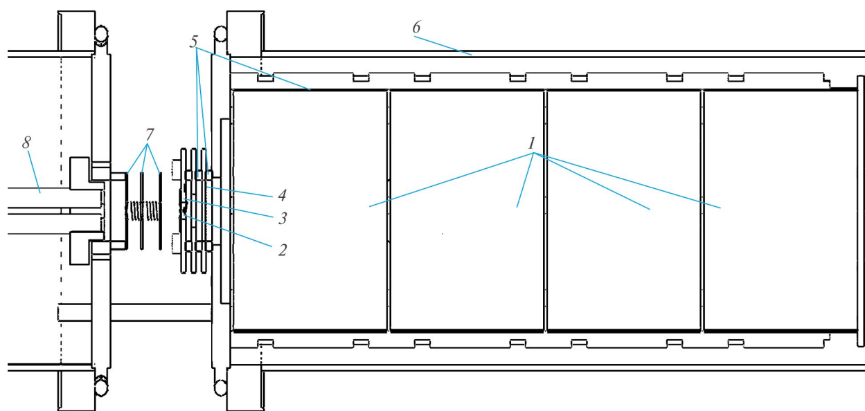
Рис. 1. Ионный источник, сочлененный со схемой формирования ионного пучка: 1 — фольги с ^{233}\text{U} в газовой ячейке, 2 — электронный эмиттер, 3 — катод, 4 — дополнительный электрод, 5 — керамические изоляторы, 6 — газовая ячейка, 7 — транспортные электроды со статическим потенциалом, 8 — электроды с радиочастотным квадрупольным потенциалом.
