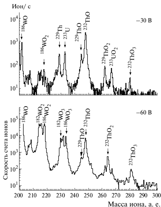
Рис. 6. Скорость счета ионов, измеренная при различных потенциалах катода и постоянной температуре эмиттера.
