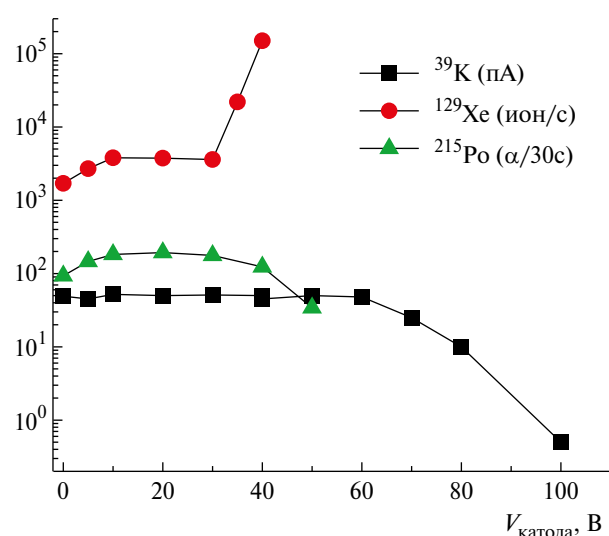
Рис. 5. Зависимости количества ионов ^{39}\text{K} , счета ионов ^{129}\text{Xe} и альфа-частиц из распада ^{215}\text{Po} от напряжения на катоде ячейки. Данные получены при давлении 50 Торр.
