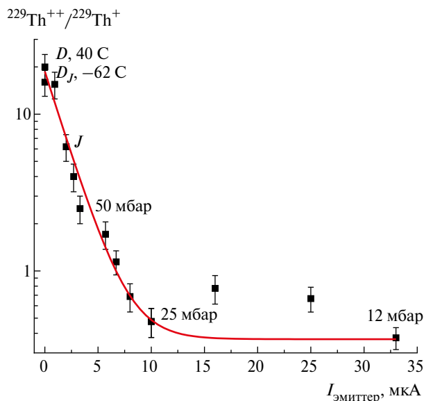
Рис. 7. Отношение скоростей счета двух- и однозарядных ионов ^{229}\text{Th} в зависимости от тока эмиттера.
