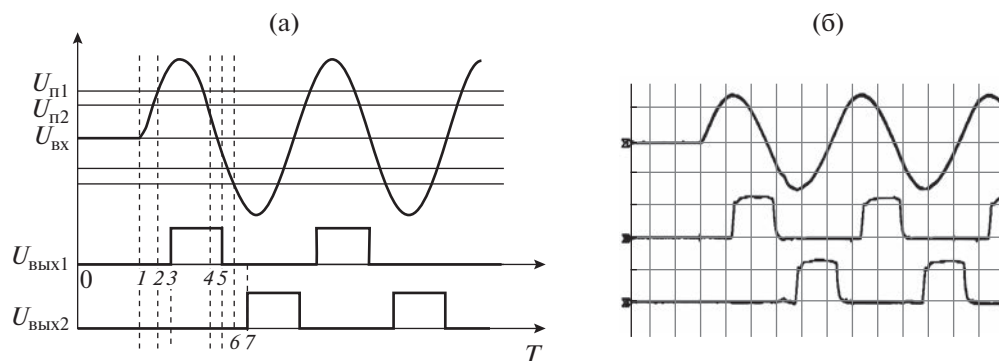
Рис. 6. Временные диаграммы формирования импульсов управления выходными ключами. а – входной сигнал U_{вх} ( U_{п1} – уровень отпираания оптрона микросхемы IC_1 , U_{п2} – уровень запираания оптрона микросхемы IC_1 ), выходное напряжение U_{вых1} микросхемы IC_1 , выходное напряжение U_{вых2} микросхемы IC_2 ; цифрами обозначены моменты времени: 1 – начало входного сигнала, 2 – момент отпираания оптрона микросхемы IC_1 , 3 – передний фронт импульса выходного напряжения микросхемы IC_1 , 4 – момент запираания оптрона микросхемы IC_1 , 5 – задний фронт импульса выходного напряжения микросхемы IC_1 , 6 – момент отпираания оптрона микросхемы IC_2 , 7 – передний фронт импульса выходного напряжения микросхемы IC_2 . б (сверху вниз) – осциллограммы входного сигнала, выходного напряжения микросхемы IC_1 , выходного напряжения микросхемы IC_2 .
