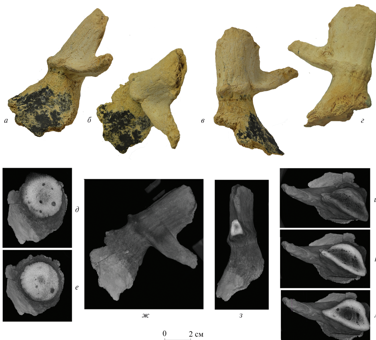
Рис. 1. Damapontica sp. nov., голотип ПИН, № 5644/3380, часть левой лобной кости с основанием рога: a — спереди, б — сверху, в — с медиальной стороны, г — с латеральной стороны; д–л — томография: 3D модели, спереди ( ж ), сверху ( и ), с поперечными сечениями розетки ( д ), пенька ( е ), первого отростка ( з ), ствола ниже облома ( к ) и у первого разветвления ( л ); Крым, пещера Таврида; нижний плейстоцен.
