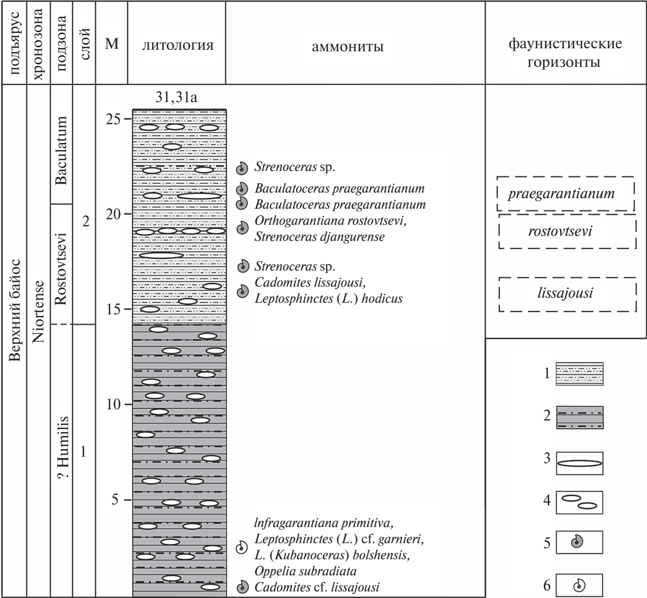
Рис. 3. Разрез байоса на левобережье р. Кыфар, местонахождения №№ 31 и 31а (по: Mitta, 2021, с изменениями и дополнениями). Обозначения: 1 – глины алевро-песчанистые, 2 – глины аргиллитоподобные, 3 – линзы, 4 – конкреции; 5, 6 – уровни находок аммонитов: 5 – в автохтонном захоронении, 6 – в переотложенных конкрециях.
