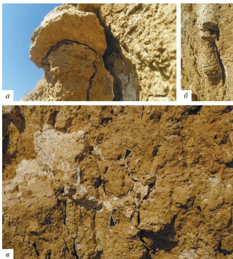
Рис. 3. Характер сохранности ископаемых нор местонахождения Сопатый Курган (сочетание обызвествленных и необызвествленных участков заполнителя): а — карбонатная корка на верхней поверхности хода, снизу заполнитель не обызвествлен; б — вложенные обызвествленные корки; в — необызвествленное ядро, окруженное карбонатной коркой.
