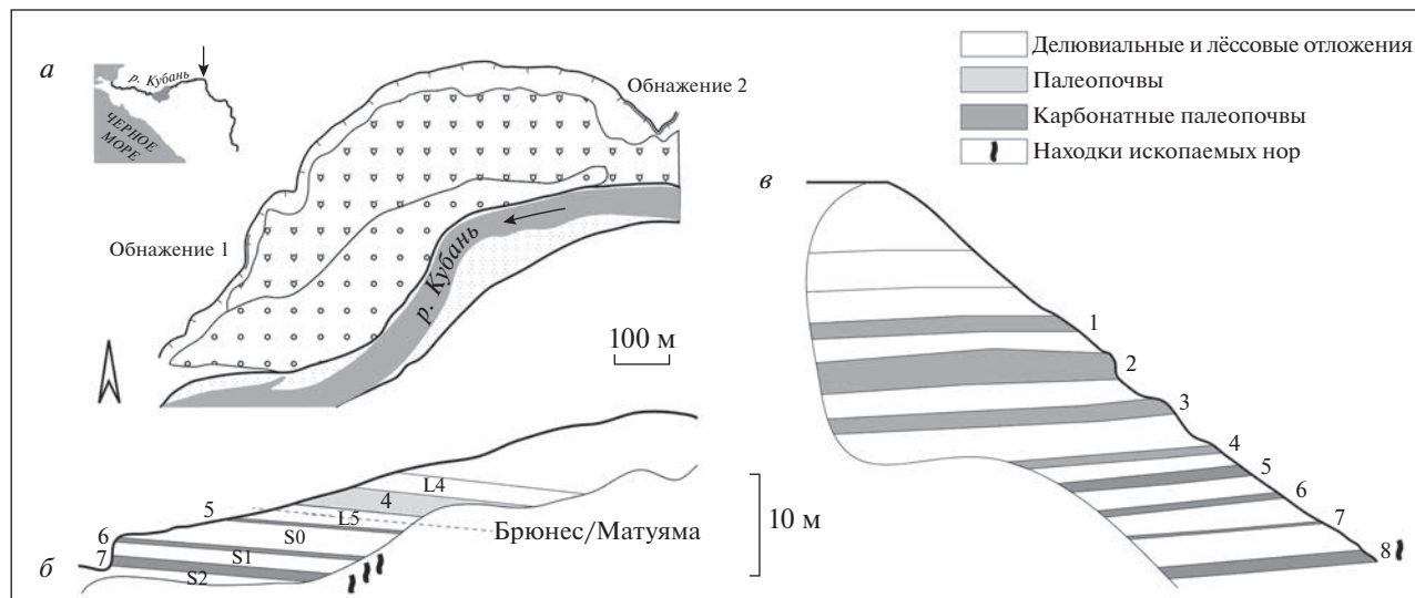
Рис. 1. Геологический разрез в районе местонахождения Сопатый Курган: а — план местности; б — обнажение 1, вид на юго-запад (цифры обозначают номер погребенной почвы от поверхности; S — нелессовидные осадки; L — лессовидные суглинки; прерывистая линия обозначает палеомагнитную границу Брюнес-Матуйма); в — обнажение 2, вид на северо-северо-запад (цифры обозначают номер погребенной почвы от поверхности).
