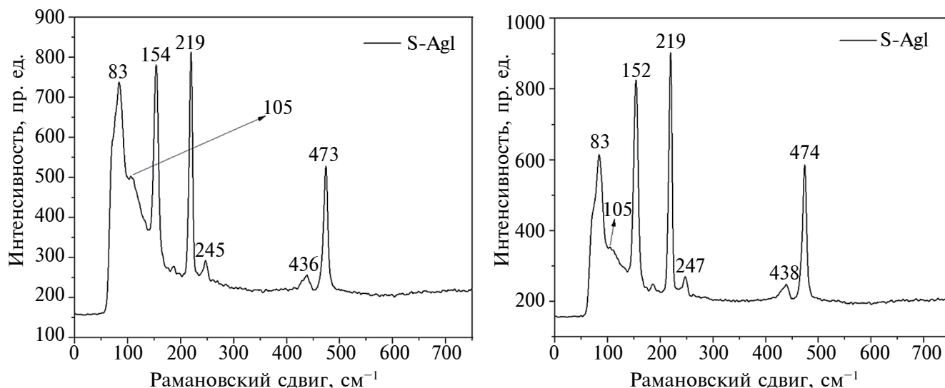
Рис. 6. Данные КР-спектроскопии для нанокomпозитов S*/AgI, приготовленных механохимической перекристаллизацией с добавками 5 мл (а) и 1 мл (б) ДМСО.
