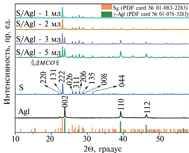
Рис. 9. Результаты РФА образцов нанокмпозитов S*/AgI, полученных на мельнице Пульверизетте 5 с добавками 1, 2, 3 и 5 мл ДМСО.
