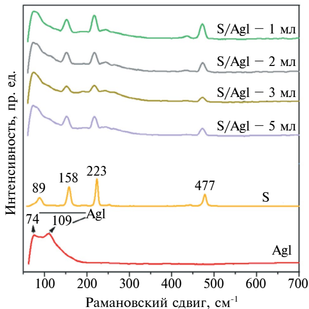
Рис. 10. Данные КР-спектроскопии для нанокмпозитов S*/AgI, полученных на мельнице Пульверизетте 5 с добавками 1, 2, 3 и 5 мл ДМСО.
