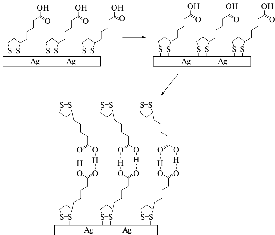
Рис. 4. Схема самоорганизации адсорбционных слоев L_2 на поверхности серебра.
