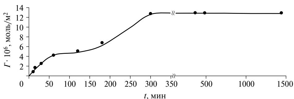
Рис. 3. Кинетика адсорбции L_2 на поверхности серебра.
