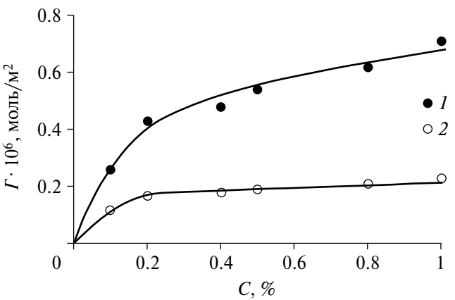
Рис. 5. Изотерма адсорбции ПДАДМАХ на поверхности полистирола до (1) и после (2) промывания в воде.
