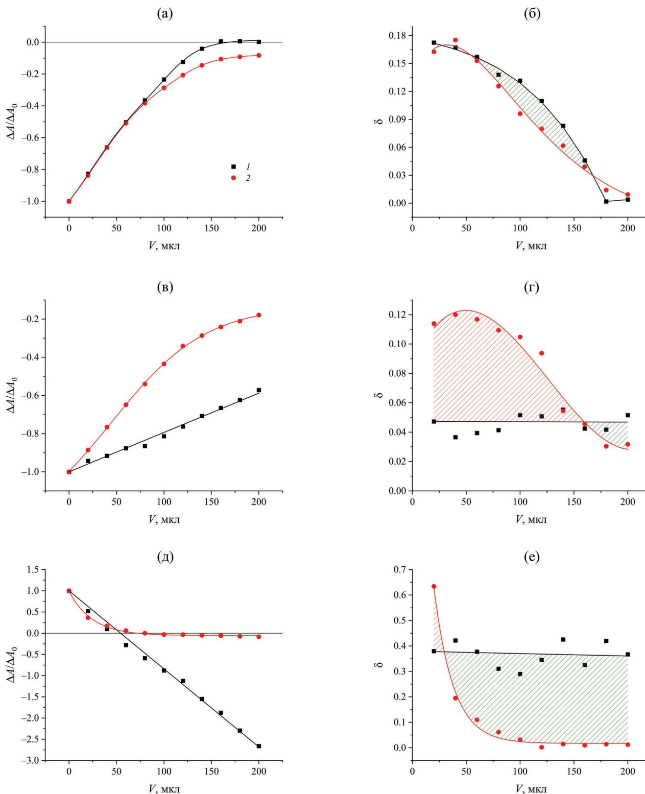
Рис. 7. Зависимости пиковой интенсивности КД-полосы, нормированной на абсолютное значение амплитуды сигнала для соответствующего контрольного образца (а, в, д), и рассчитанных значений \delta (б, г, е) от вносимого объема дистиллированной воды (1) и гидрозоля НЧЗ (2) в ЖКД ДНК с разным содержанием ПЭГ (масс. %): 15 (а, б), 21 (в, г), 27 (д, е). Стандартные отклонения, рассчитанные по трем независимым измерениям, не превышают 7% (а, в, д) и 14% (б, г, е).
