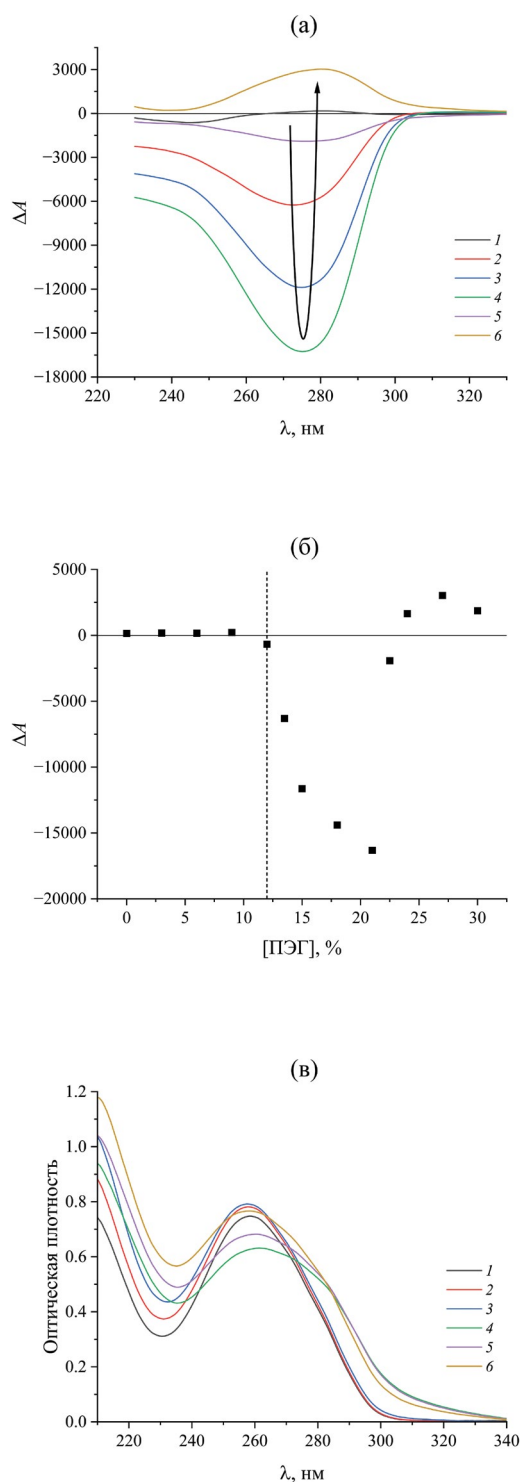
Рис. 4. (а) Спектры КД систем с различным содержанием ПЭГ (масс. %): 1 – 0, 2 – 13.5, 3 – 16.5, 4 – 21, 5 – 22.5, 6 – 27. (б) Зависимость амплитуды КД-сигнала от концентрации ПЭГ в системе. Стандартные отклонения, рассчитанные по трем независимым измерениям, не превышают 7%. (в) Спектры поглощения систем с различным содержанием ПЭГ (масс. %): 1 – 0, 2 – 6, 3 – 12, 4 – 18, 5 – 24, 6 – 30.
