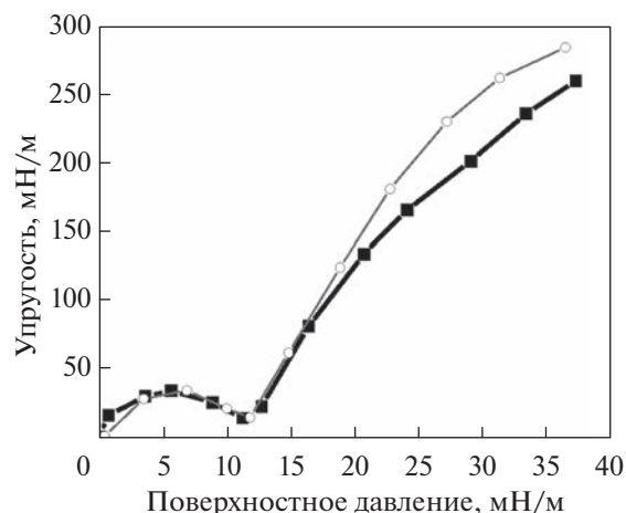
Рис. 5. Зависимости динамической упругости от поверхностного давления для монослоя ДПФХ на растворе ПДАДМАХ 0.2 мас. % (пустые круги), на буфере (закрашенные квадраты) при T = 25^\circ\text{C} .
