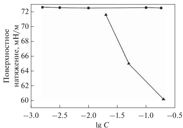
Рис. 4. Зависимости поверхностного натяжения от десятичного логарифма концентраций полиэлектролита (мас. %) ПСС (треугольники), ПДАДМАХ (круги) при T = 25^\circ\text{C} .
