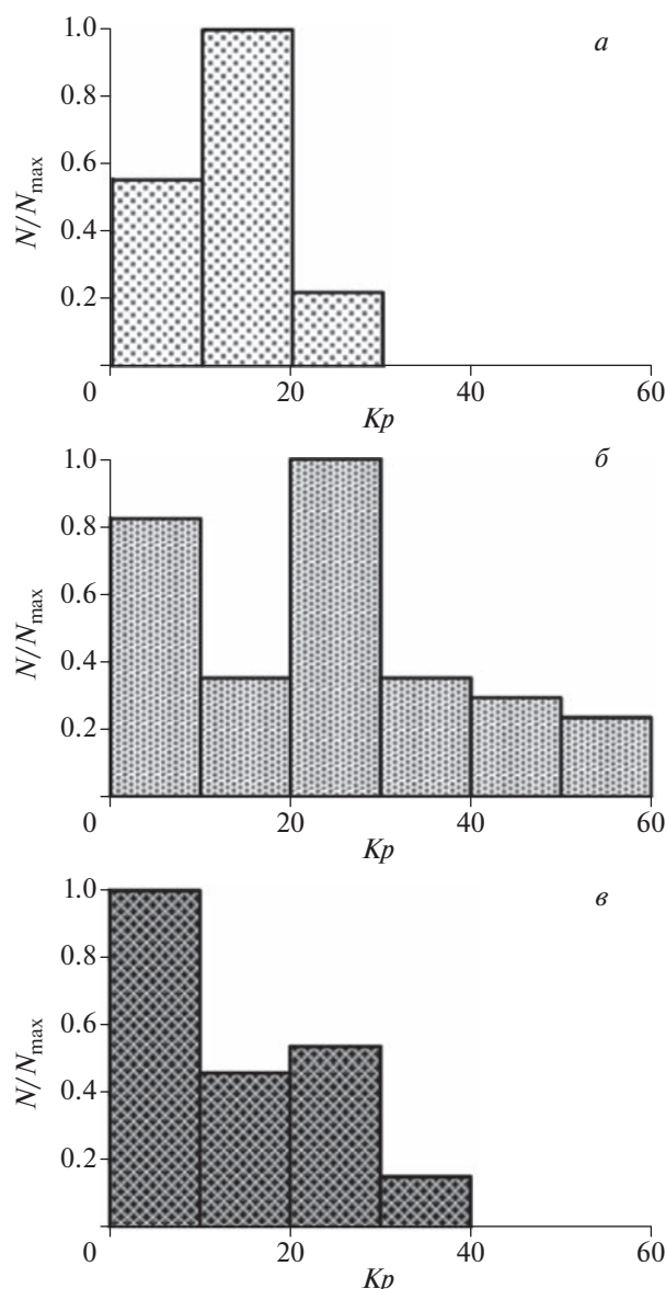
Рис. 5. Зависимость частоты наблюдения серий Pc1 от геомагнитной активности ( K_p -индекса), регистрируемых в BOX и MND: (а) — одновременно; (б) — с западным дрейфом; (в) — с восточным дрейфом.
