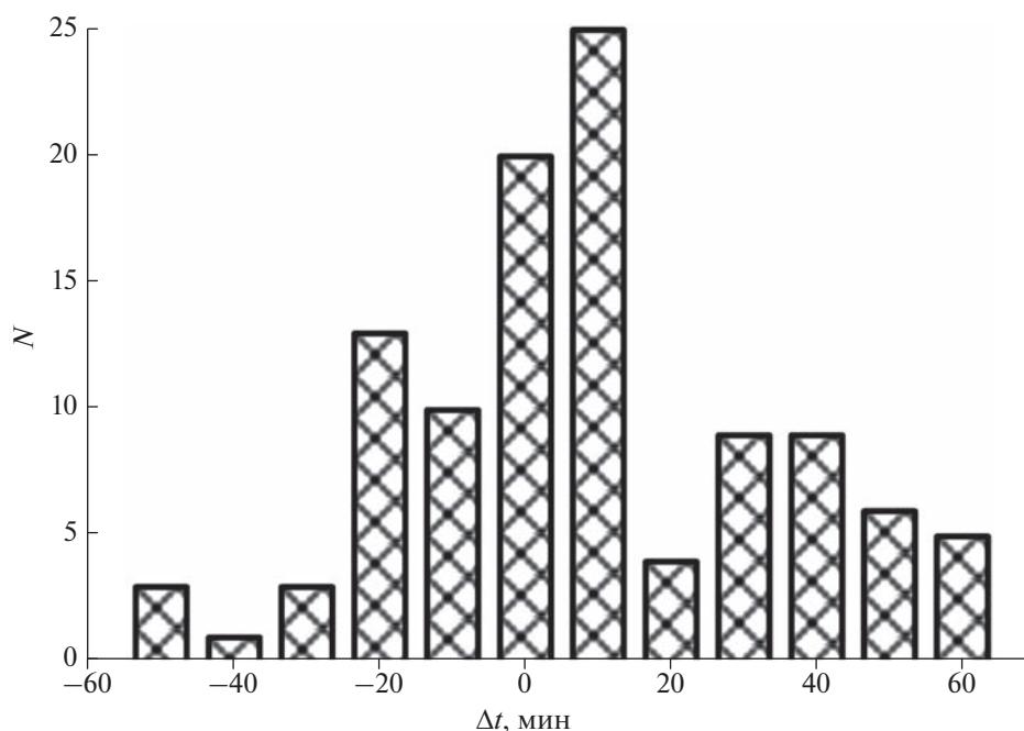
Рис. 3. Зависимость числа наблюдений серий Pc1 от временного интервала между началом пульсаций в BOX по отношению к MND.
