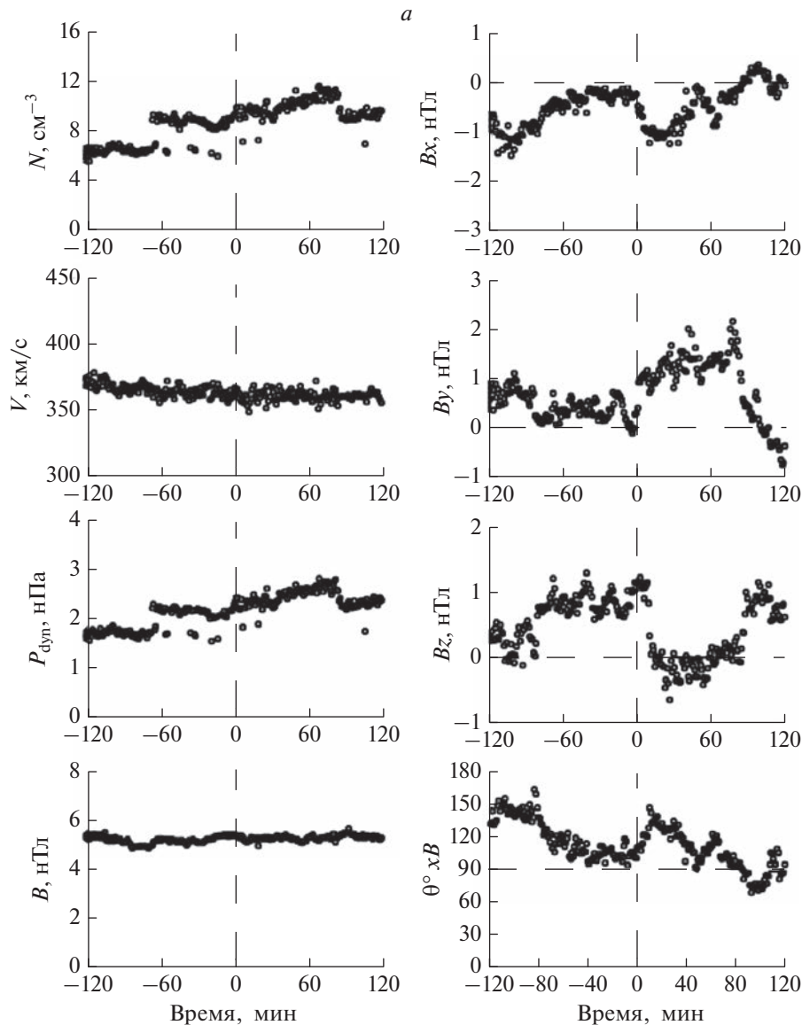
Рис. 6. Динамика параметров солнечного ветра и ММП, полученная методом наложения эпох для случаев начала (а) — одновременного наблюдения; (б) — запаздывания; (в) — опережения серий Pc1 в BOX по отношению к MND.
