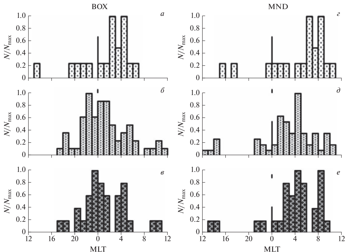
Рис. 4. Суточная вариация числа случаев Pc1 , наблюдаемых в BOX и MND, (a, d) — одновременно; (б, е) — с западным дрейфом; (в, е) — с восточным дрейфом.
