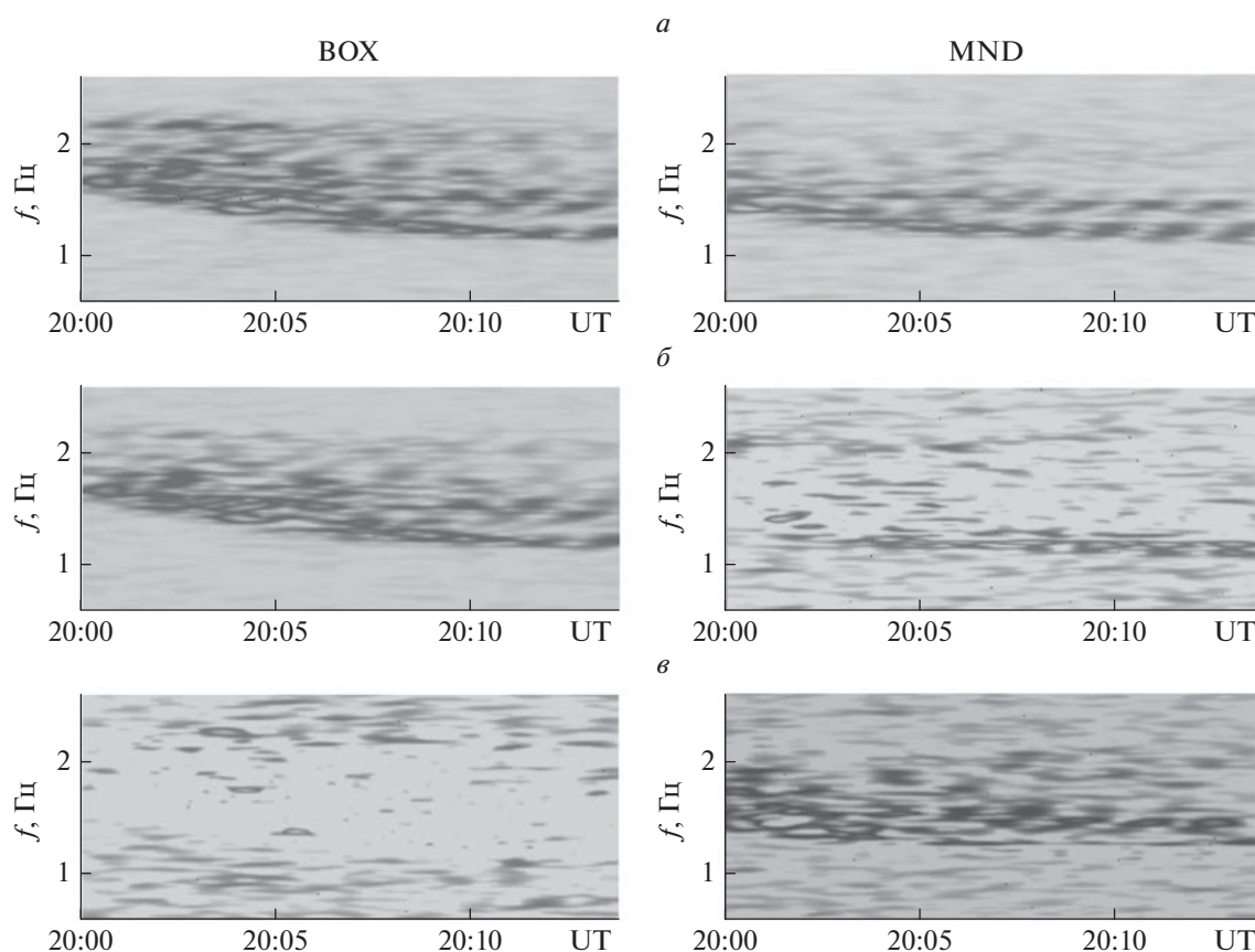
Рис. 7. Пример определения типа поляризации пульсаций Pc1 , наблюдаемых одновременно в BOX и MND 24.02.1999 г.: (a) — полная спектральная плотность, (б) — спектральная плотность левополяризованной и (в) — правополяризованной моды исходного сигнала.
