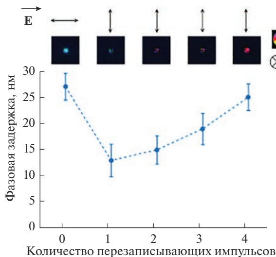
Рис. 2. Зависимость фазовой задержки от количества перезаписывающих импульсов и соответствующие псевдоцветовые карты, ориентации медленной оси двулучепреломления модифицированных областей НПС: \vec{k} — направление распространения записывающего пучка, \vec{E} — плоскость поляризации лазерного пучка.
